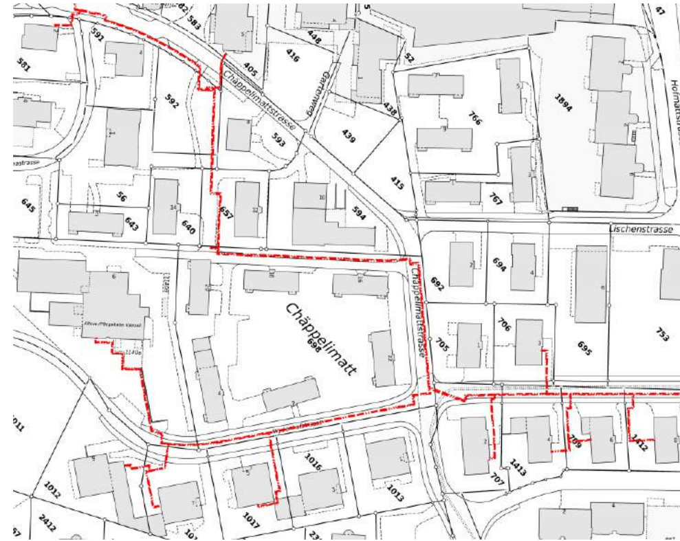
Fernwärmeplan 2020
